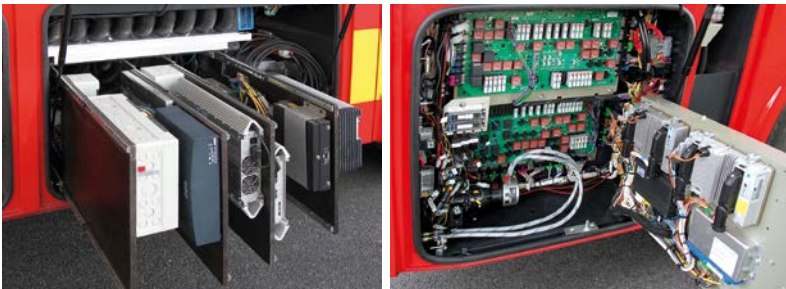
Einbau und Anschluss der Steuerungskomponenten
